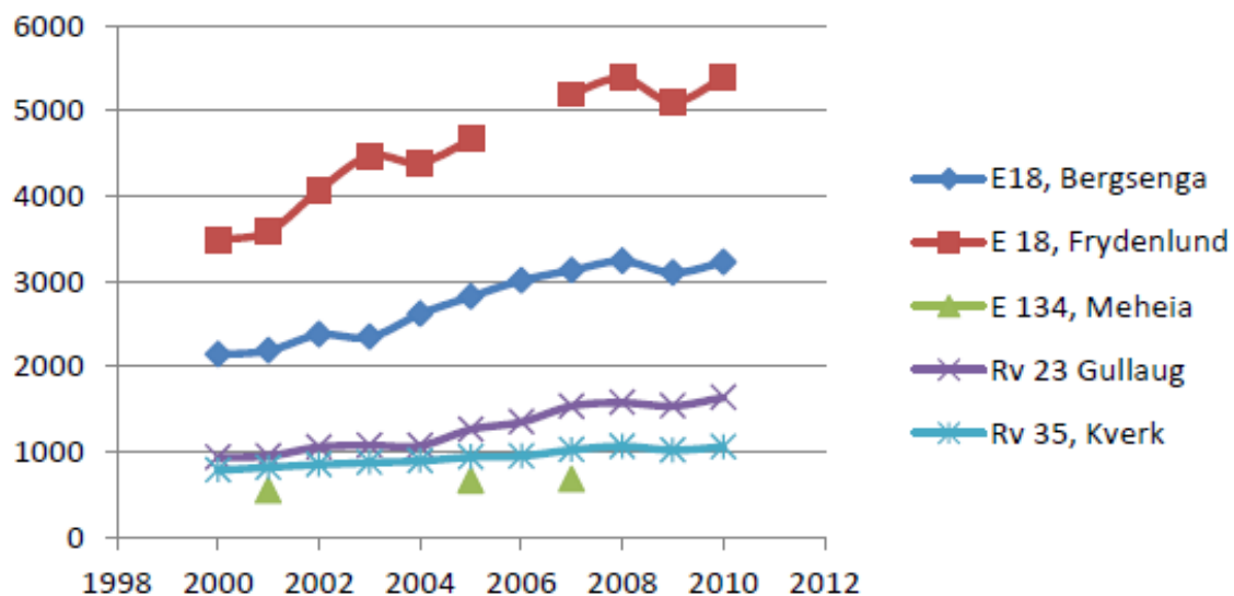
ÅDT tungtransport i hovedinnfartsårer til Buskerudbyen.
