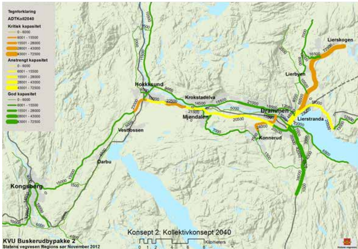
Trafikbelastning på vegnettet i kollektivkonseptet i 2040.
