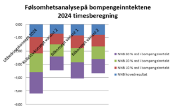
Følsomhetsanalyse for bompengeinntektene i 2024.
