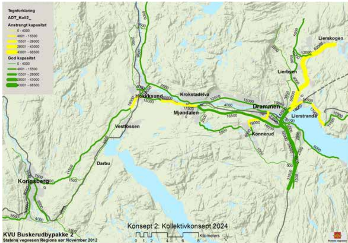
Trafikbelastning på vegnettet i kollektivkonseptet i 2024.
