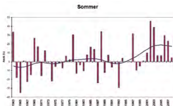
Figur 4.7.2 Avviket fra normalperioden i års- og sesongavviken- ning i Nigardsjøen 1963–2008
