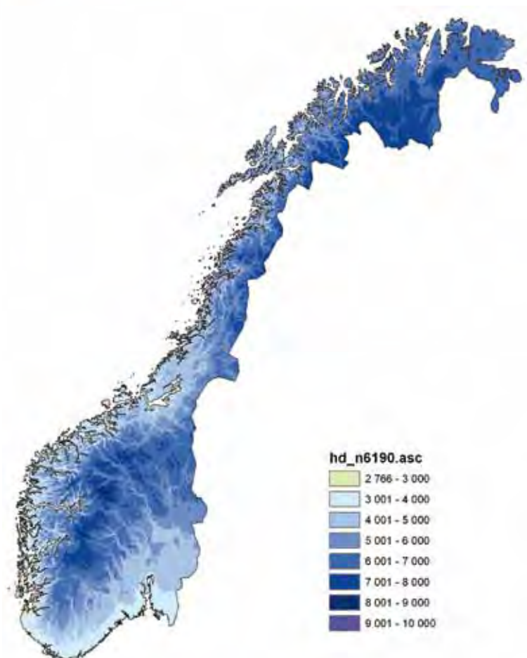
Figur 2.2.5 Fyringsgraddagsum i normalperioden 1961–90
