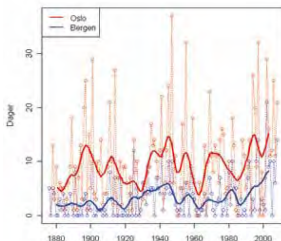
Figur 3.1.6 Varme døgn 1870–2008: Antall døgn per år med døgnmiddeltemperatur over 20^{\circ}\text{C} i Oslo og Bergen
