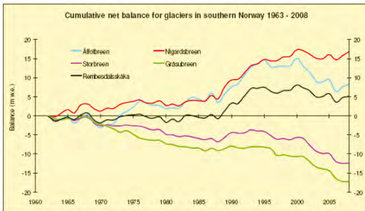
Figur 4.7.3 Kumulativ nettobalanse for breer i Sør-Norge 1963–2008 (Kjølmoen, 2009).
