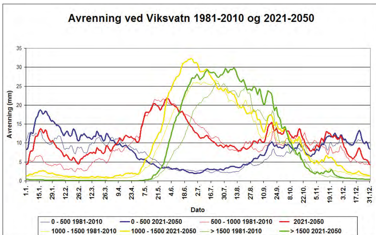
Figur 5.3.4 Sesongfordeling av avrenningen i kontrollperiode og scenarioperiode for fire høydesoner i feltet til Viksvatn i Gaular i Sunnfjord.
