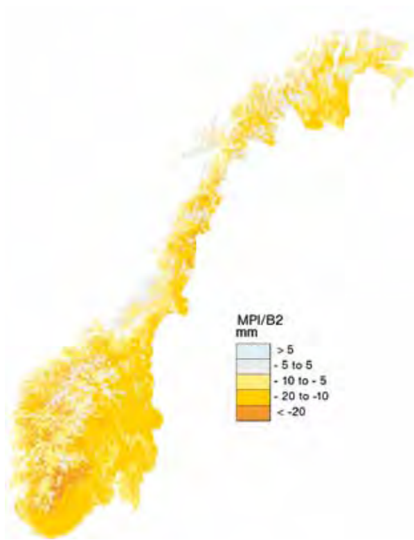
Figur 5.3.9 Endring i maksimalt markvannsunderskudd i kort og lang framskrivningsperiode.
