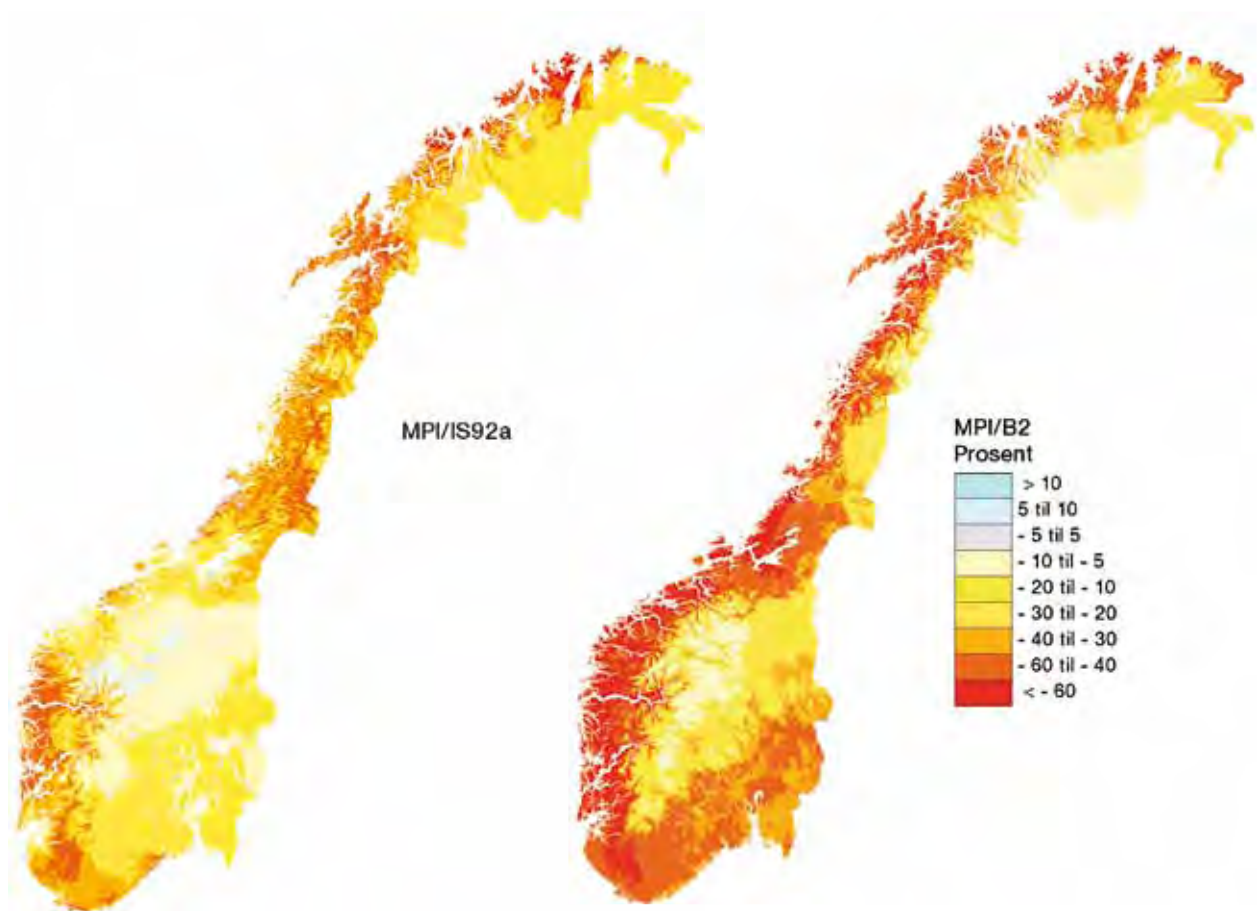
Figur 5.3.6 Endring i maksimal årlig vannekvivalent av snømagasinet for kort og lang framskrivningsperiode. Begge framskrivingene er basert på ECHAM4-modellen, men bygger på ulike utslippsscenarioer (IS92a for kort og B2 for lang periode).
