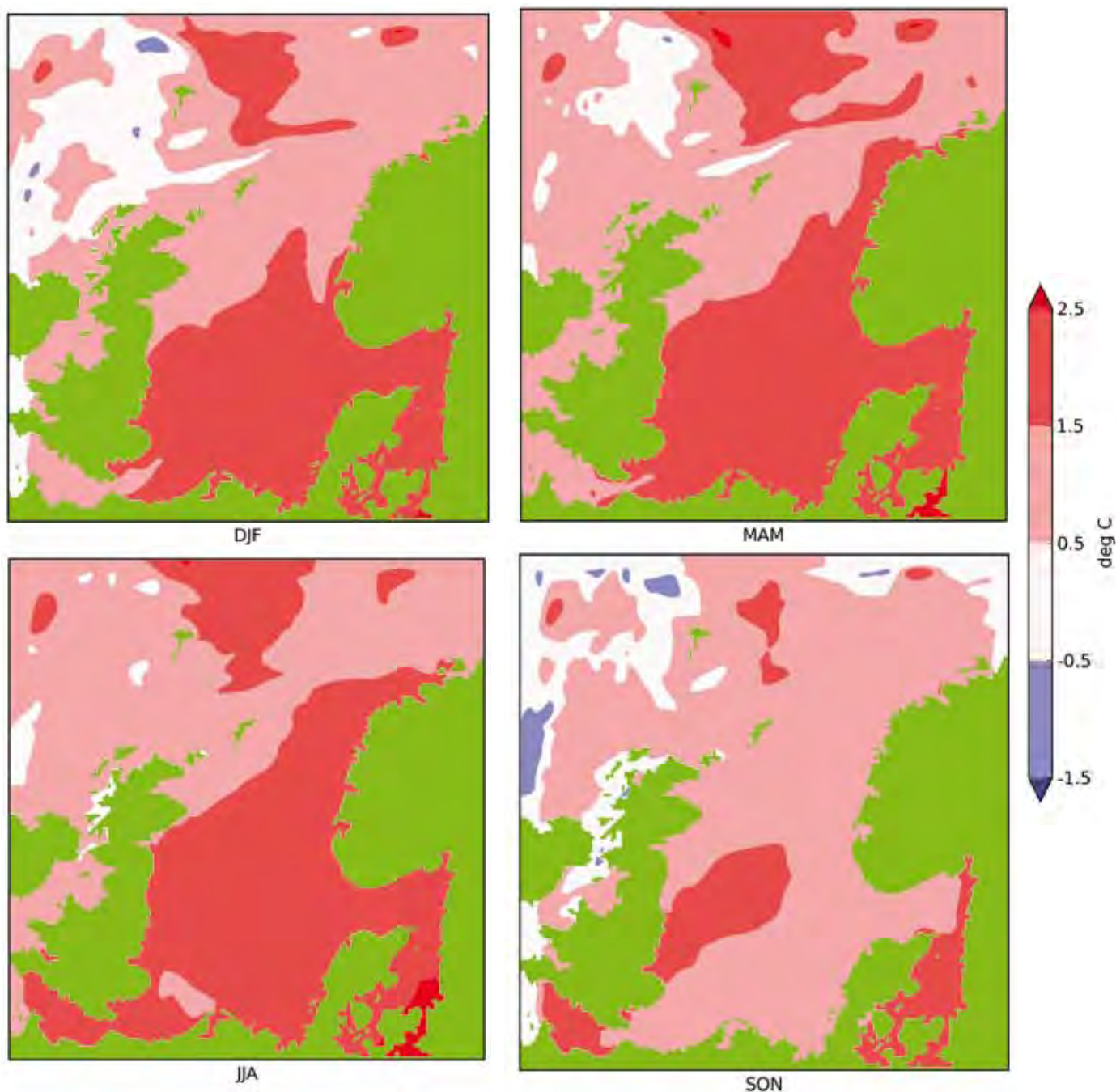
Figur 5.4.3 Endring i overflatetemperaturen i Nordsjø-nedskaleringen. Endring fra kontrollperiode 1972–97 til framtidsscenario 2072–97
