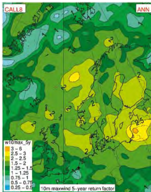
Figur 5.2.16 Estimert returfaktor rundt år 2050 for døgnlign maksimal vindstyrke i 10 meters høyde. De tre kartene er beregnet fra ulike prosentiler i kontrollperioden (dagens klima). Øverst til venstre er kart beregnet ut fra 5-prosentilen, øverst til høyre prosentilen som tilsvarer 1 gang per år, og til høyre her prosentilen som tilsvarer en gang per femte år.
