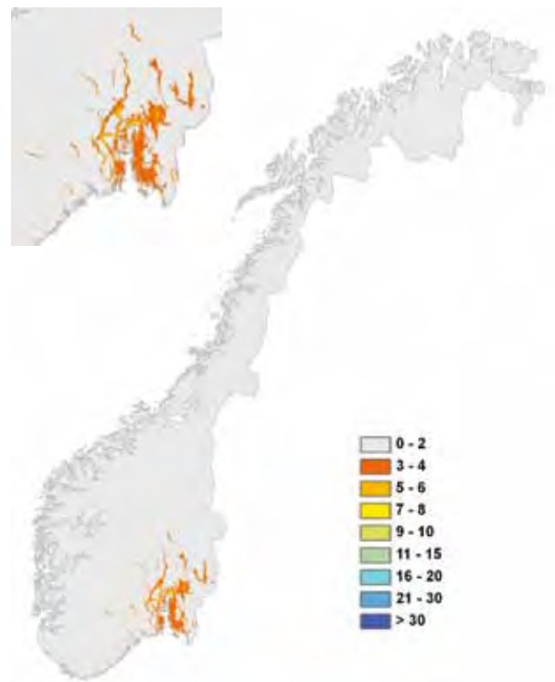
Figur 2.2.6 Midlere antall døgn med middeltemperatur over 20 °C i normalperioden 1961–90
