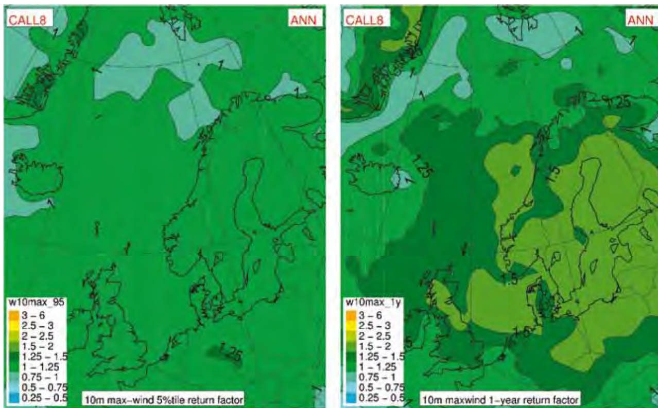
Figur 5.2.16 Estimert returfaktor rundt år 2050 for døgnlign maksimal vindstyrke i 10 meters høyde. De tre kartene er beregnet fra ulike prosentiler i kontrollperioden (dagens klima). Øverst til venstre er kart beregnet ut fra 5-prosentilen, øverst til høyre prosentilen som tilsvarer 1 gang per år, og til høyre her prosentilen som tilsvarer en gang per femte år.
