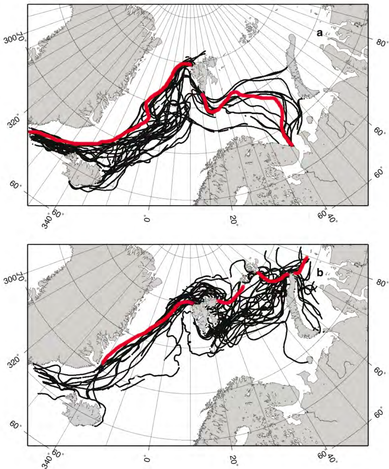
Figur 3.4.1 Iskantposisjoner for perioden 1850–1899 (svarte linjer) analysert av Divine og Dick (2006), med midlere iskant fra perioden 1979–2000 basert på satellittdata markert med rød linje. (a) viser data for april og (b) viser data for august.
