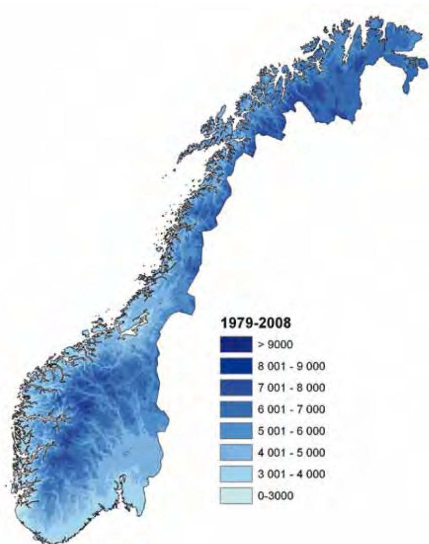
Figur 4.3.1 Fyringsgraddagsum i perioden 1979–2008
