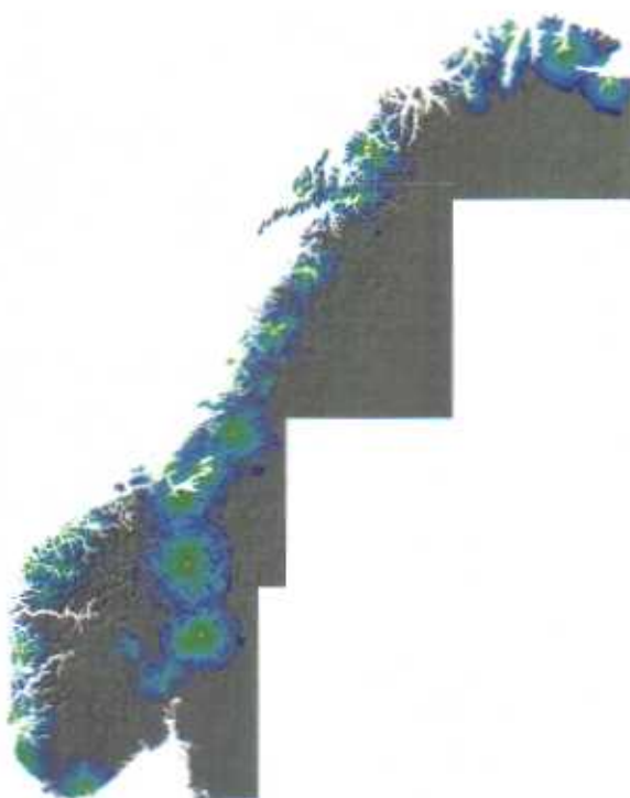
Figur 5: Dekning for MUX6 i 470-790 MHz Befolkningsdekning 51,5 prosent
