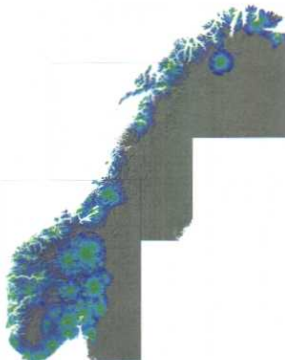
Figur 10: Dekning for én signalpakke i 790-862 MHz Befolkningsdekning 95,9 prosent
