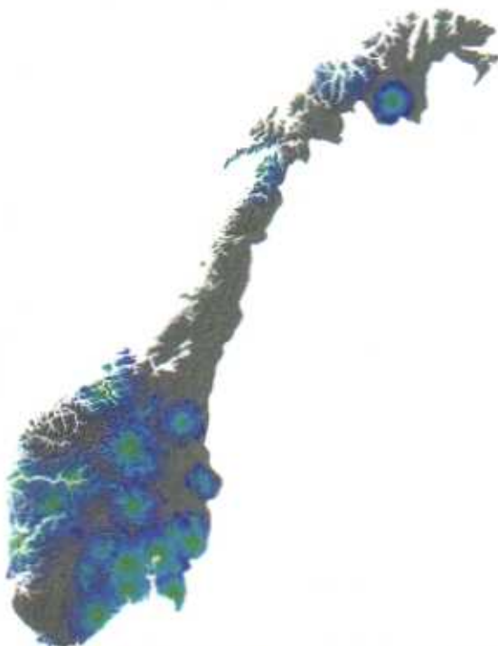
Figur 8: Dekning for MUX6 i 790-862 MHz Befolkningsdekning 61,9 prosent
